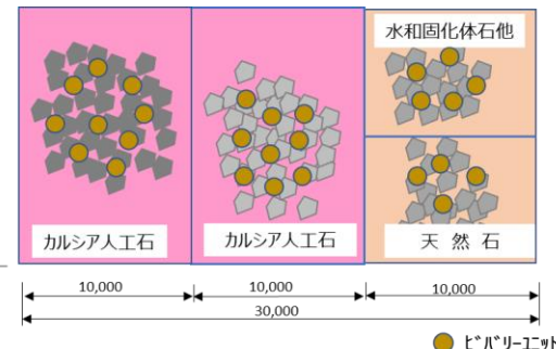
図8 基質の配置図
