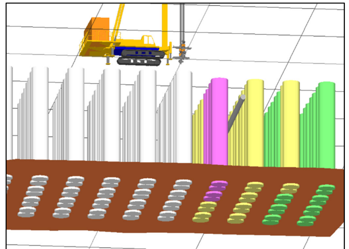
施工中以外の 3D 表示例
