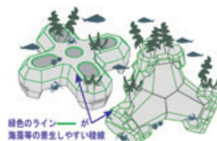
コンクリートブロックの稜線に集中して着生したコンブ科の海藻
