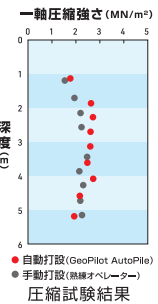
圧縮試験結果
