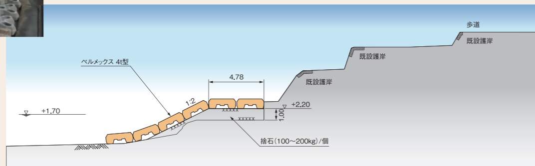
(図は4t型を用いた護岸)
