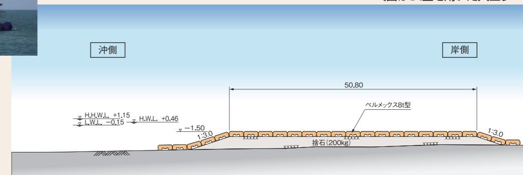
(図は8t型を用いた人工リーフ)
