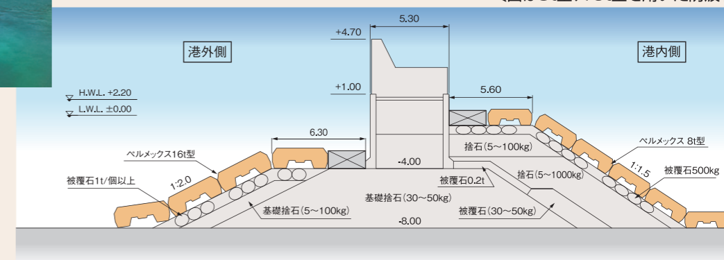
(図は8t型、16t型を用いた防波堤)
