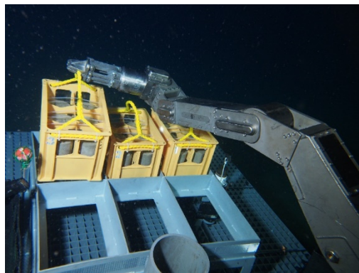
図5 「しんかい6500」により水深3,515mに運搬され、プラットフォーム上に設置された供試体の様子（写真は3つ目のプラスチック容器を設置中の様子）
