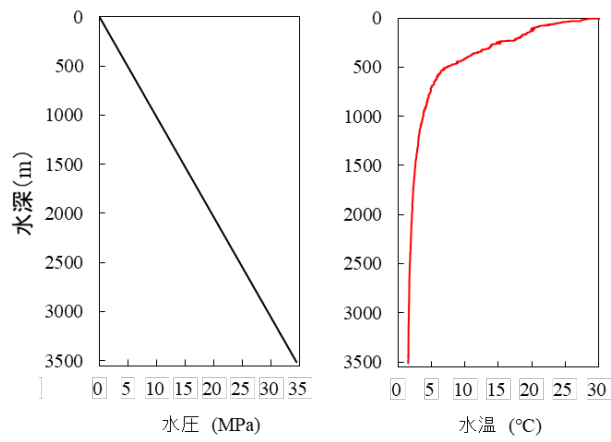
図1 水深と水圧(左)、水温(右)の分布
