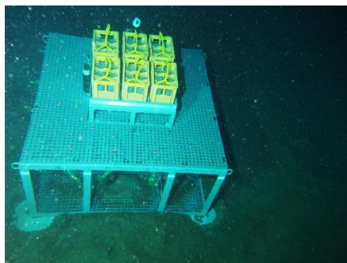
図6 プラットホーム上で曝露が開始されたコンクリート供試体
