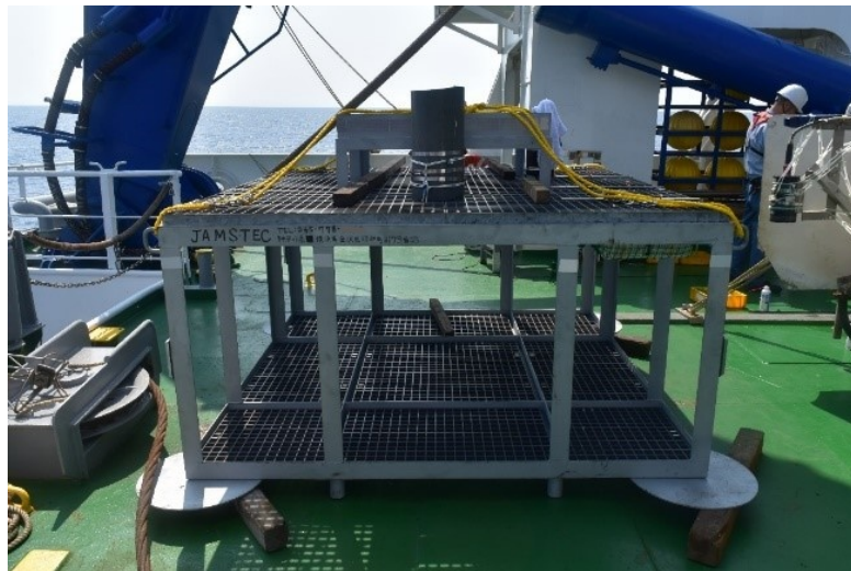
図2 コンクリート供試体を設置するためのプラットフォーム（「ディープ・トウ」と連結され深海底に運搬された）
