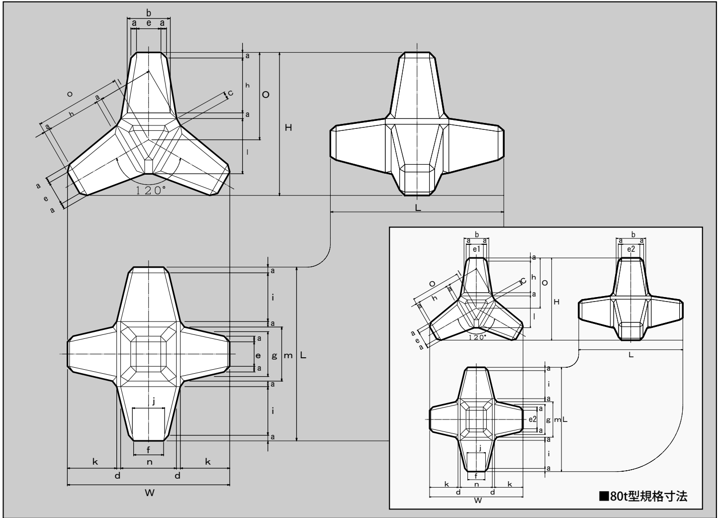
ペンタコン規格寸法表
