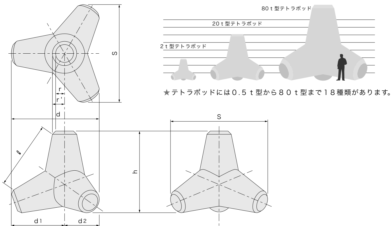
テトラポッドの寸法表
